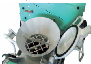
Boccaporto con valvola di sicurezza integrata per manovre agevoli e sicure
