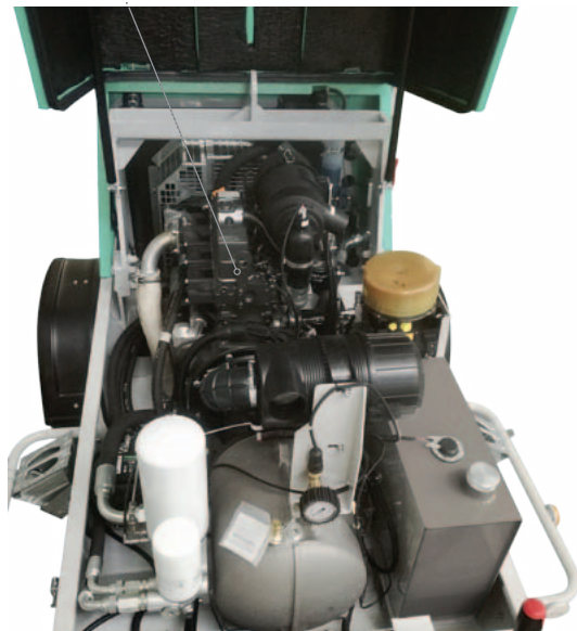
Motore diesel Yanmar - 35 kw, 4 cilindri
