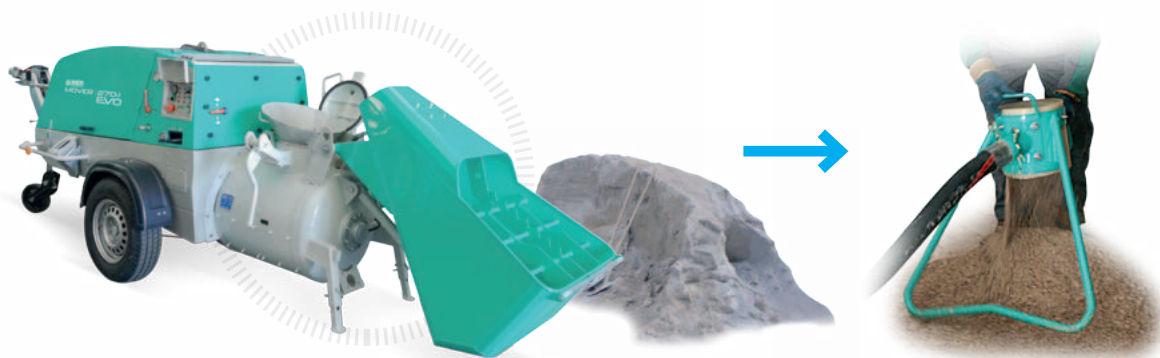
Cavalletto rompigitto
